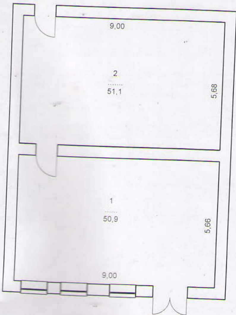
Позтажный план М 1:100
